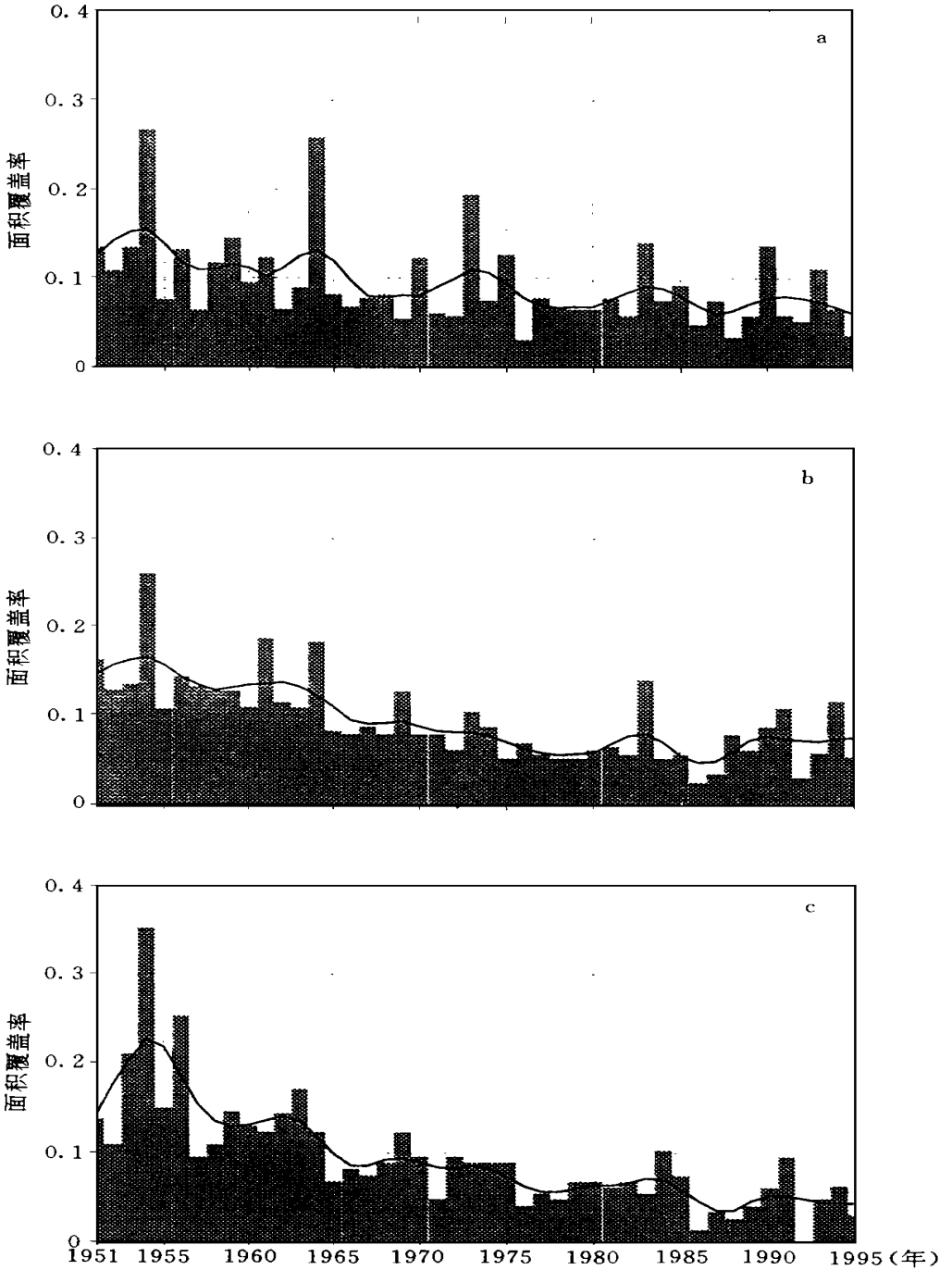
图3 1951~1995年中国最大4a中雨以上、暴雨 和大暴雨降水日数发生的面积覆盖率变化 (a. 日降水量 10 mm; b. 日降水量 50 mm; c. 日降水量 100 mm)
